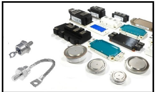
Figura 12- Distintos tipos de diodos rectificadores de potencia elevada
