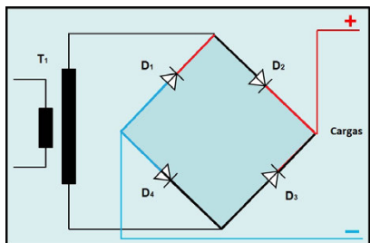
Figura 6- Puente de Graetz de conexión aclarada
