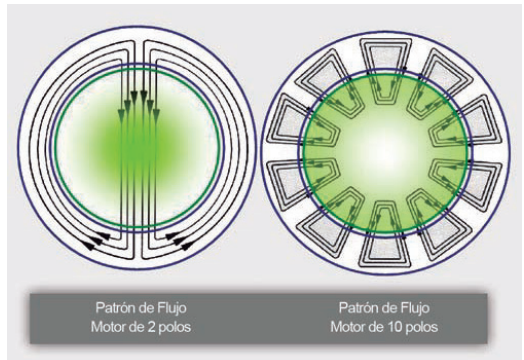
Figura 2. Patrón de flujo magnético del estator según cantidad de polos.
