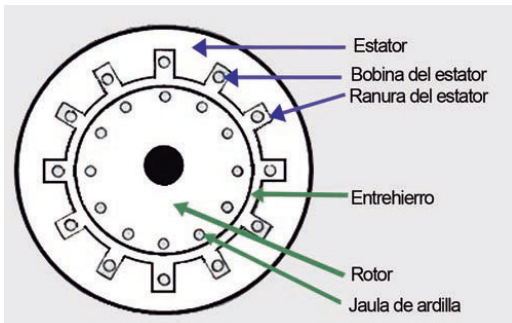
Figura 1. Ubicación del entrehierro en un motor eléctrico.
